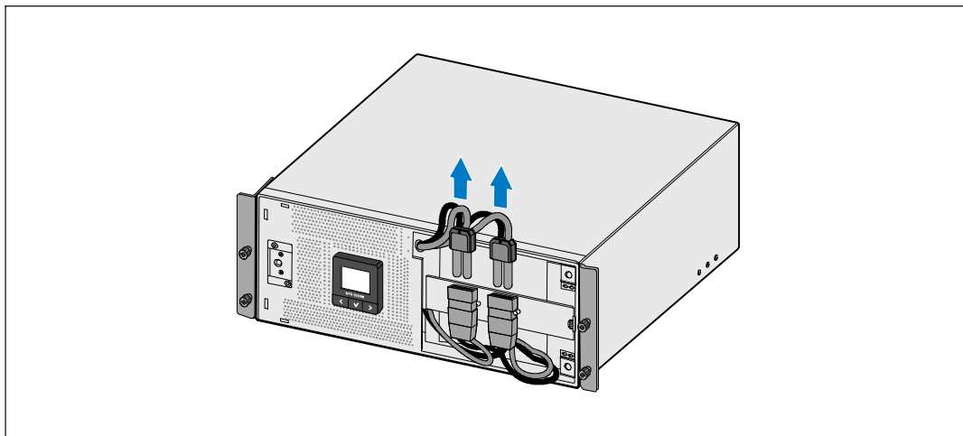
図 25. 内蔵バッテリーのコネクタの取り外し方法
