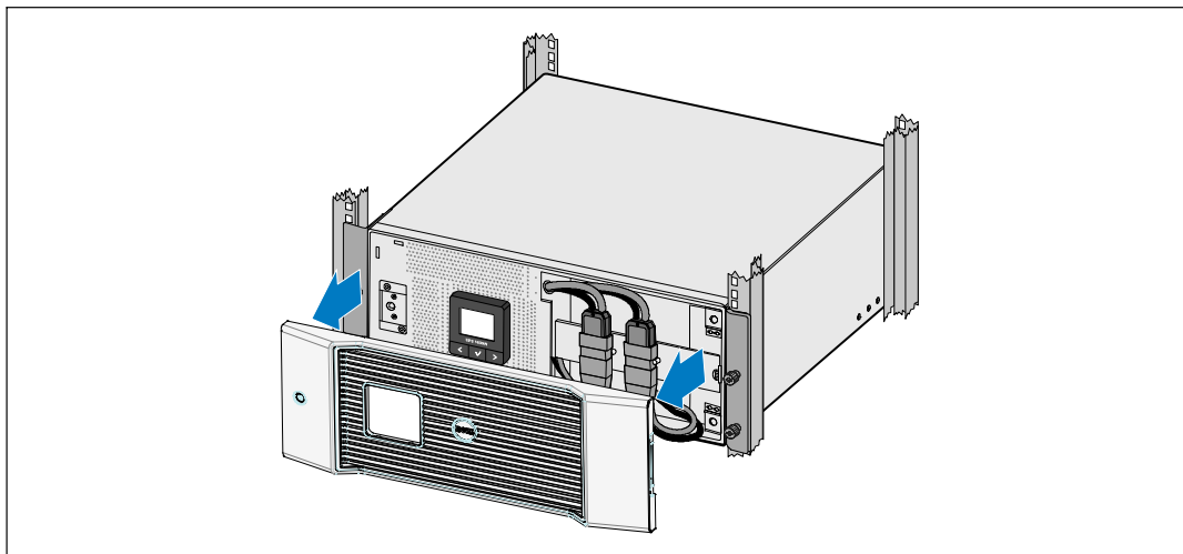
図 24. UPSのフロントカバーの取り外し方法
