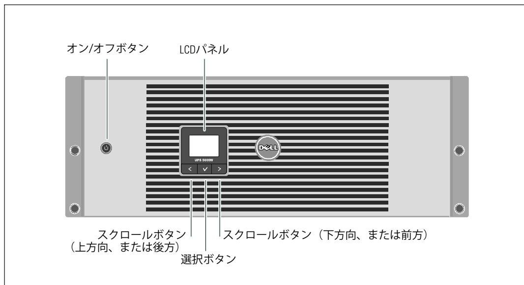
図 6. Dell ラインインタラクティブ式ラックUPS前方パネル
