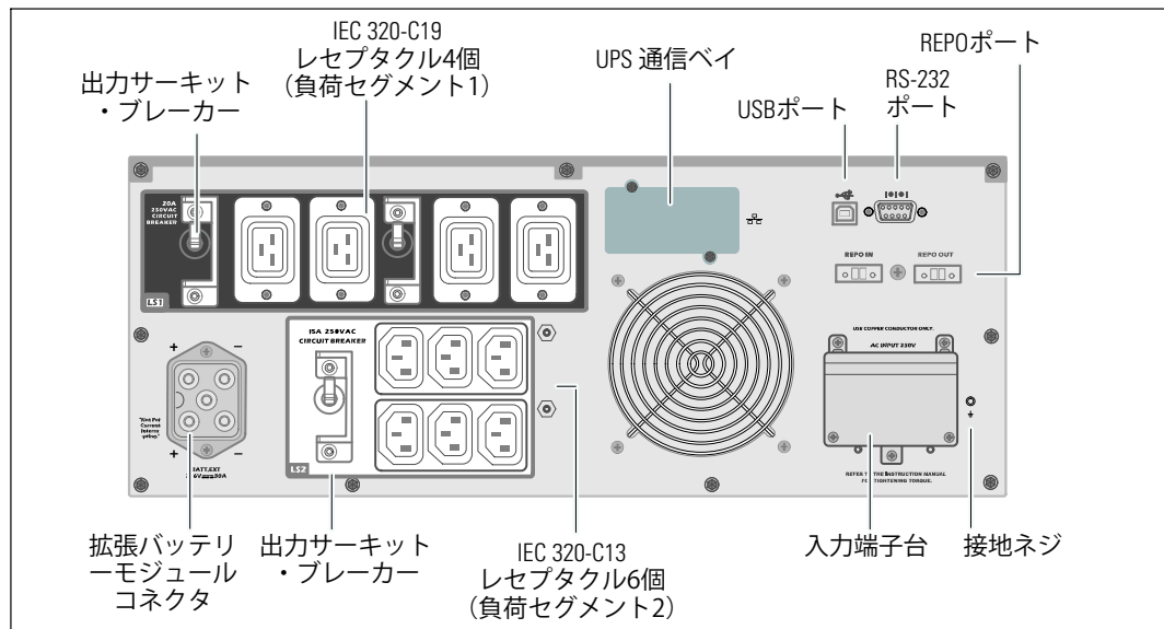
図 5. 5600W、230V 後方パネル
