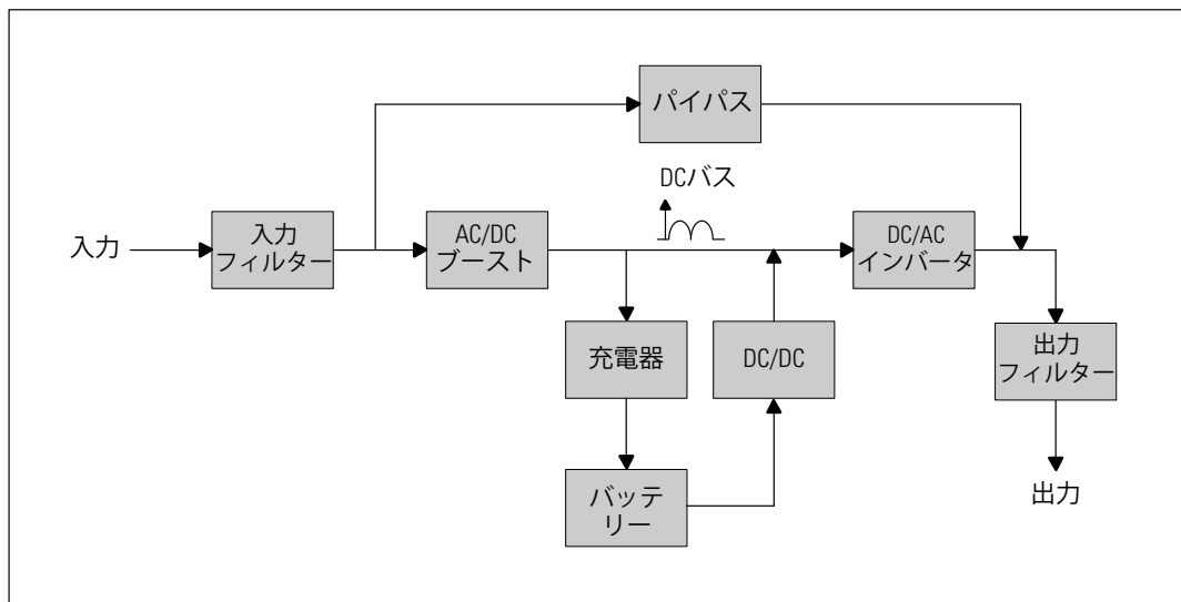
図 27. 5600Wラインインタラクティブ式UPSブロック図
